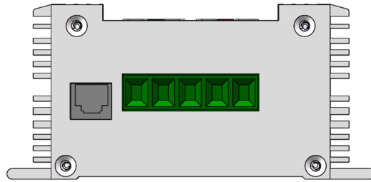
图 2-3 产品上侧连接口图
